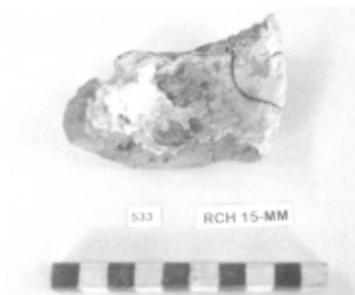
Figura 7. Fragmento de una cuchara. Se observan escorificaciones y capas de recubrimiento blanquecino.
