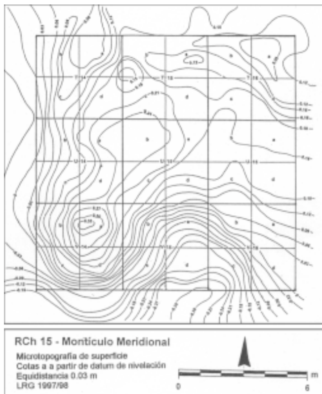
Figura 3. Planta del Montículo Meridional del sitio 15.
